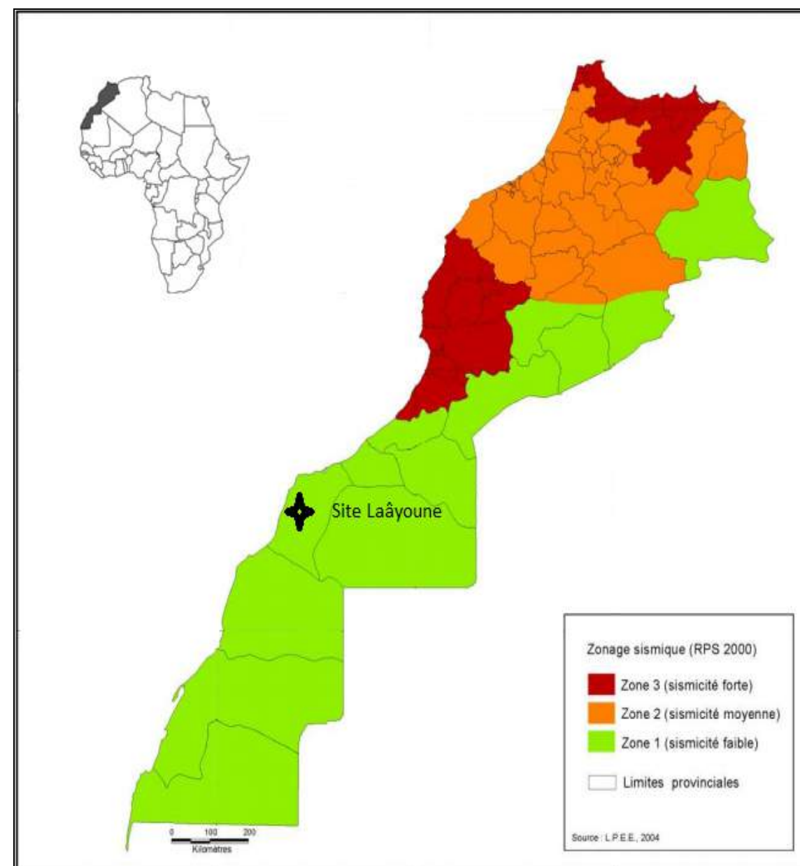
Figure 49 : Zonage sismique au Maroc (RPS 2000)
