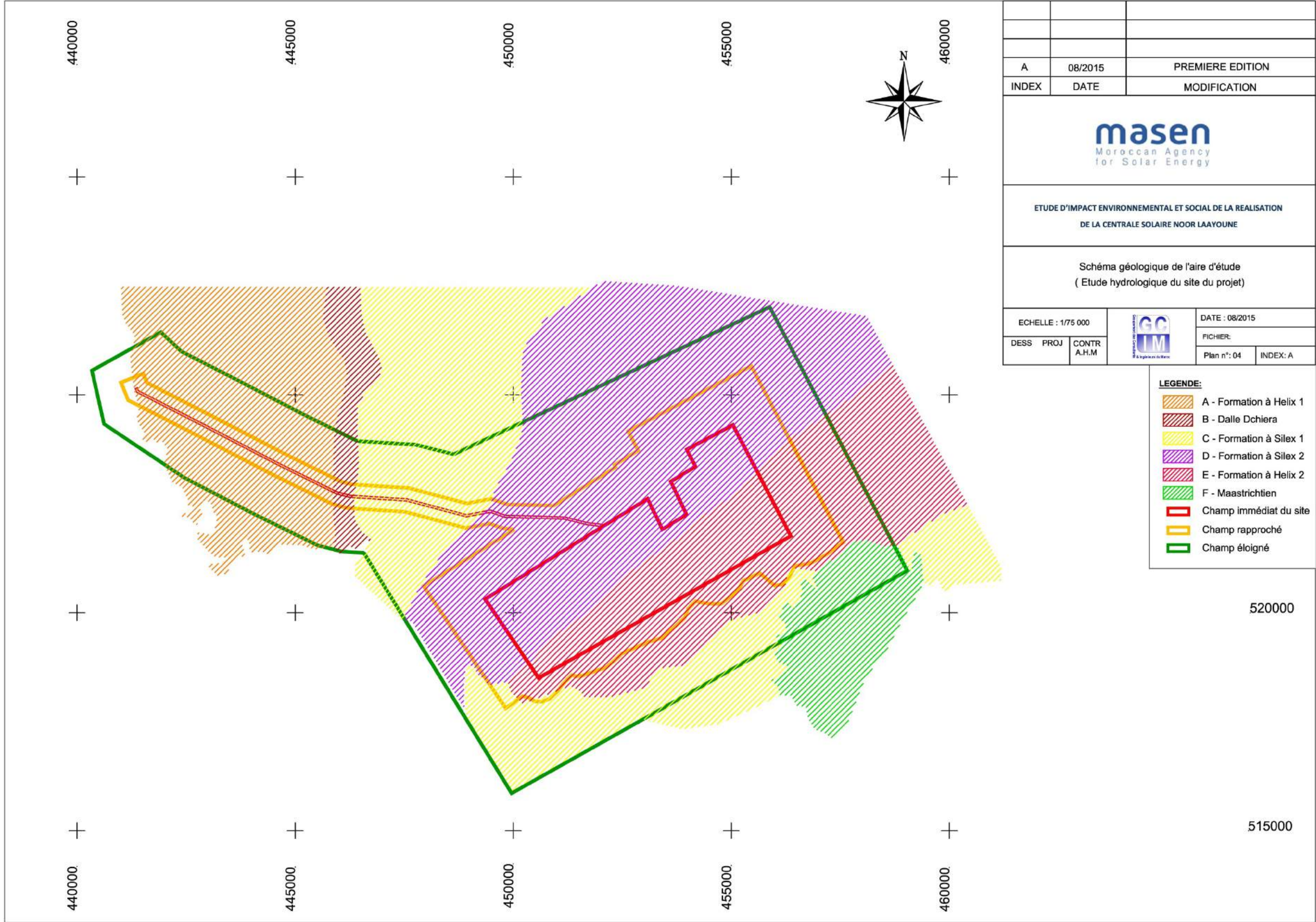
PLAN N° 4 : SCHEMA GEOLOGIQUE de la zone d'étude
