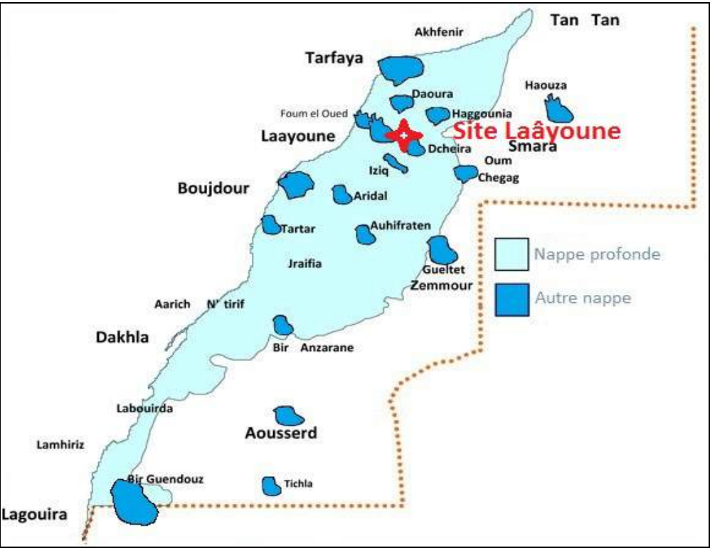
Figure 48 : Nappes d’eau du bassin Tarfaya-Laâyoune-Boujdour-Dakhla
