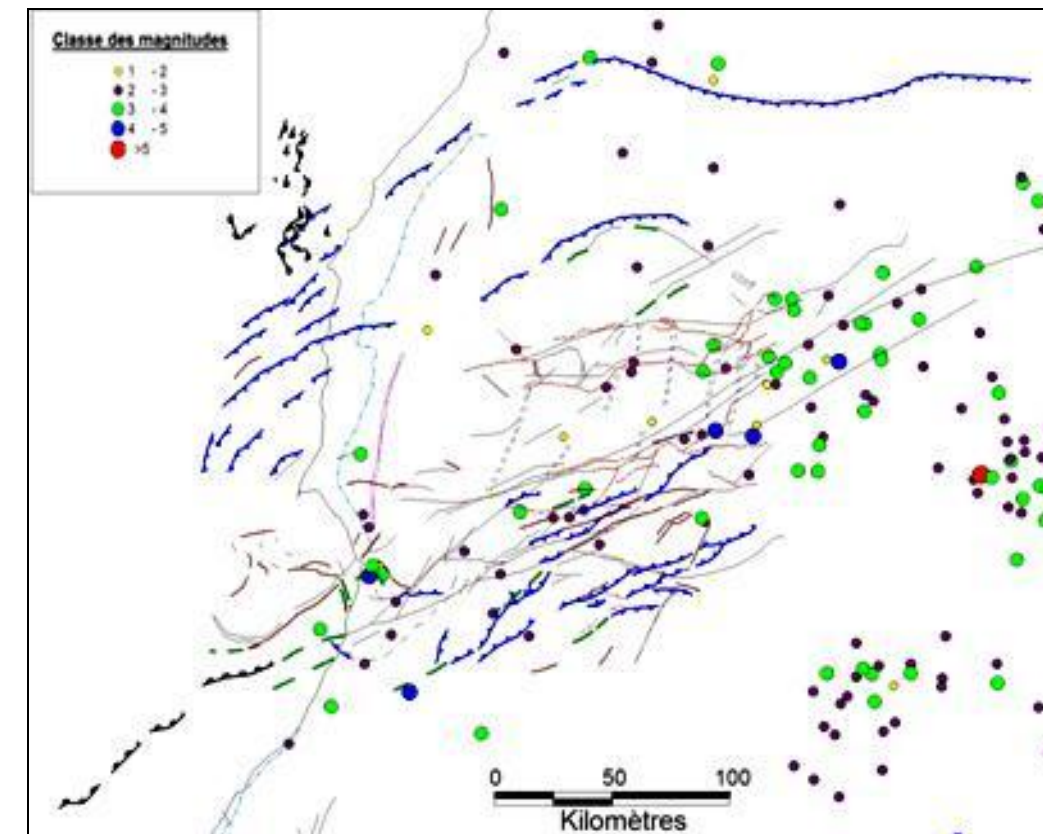
Figure 40 : Carte séismotectonique du Haut Atlas
