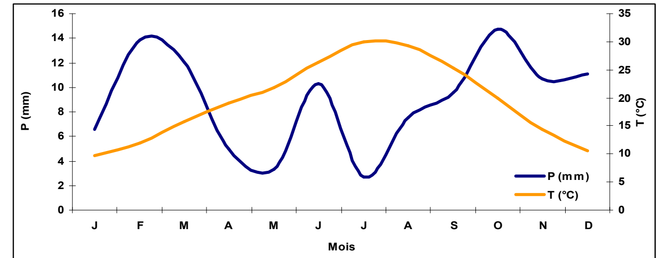
Figure 56 : Diagramme ombrothermique - Station : Mansour Ed Dahbi - Période : 1980 - 2009
