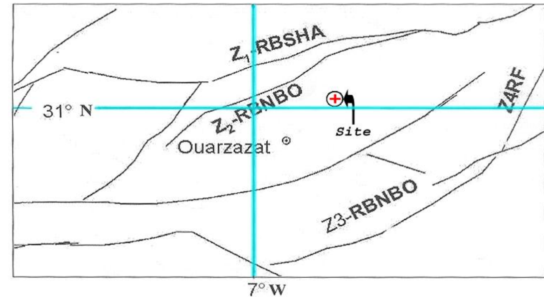
Figure 42 : Carte des principales failles à potentiel sismique dans la région d'Ouarzazate
