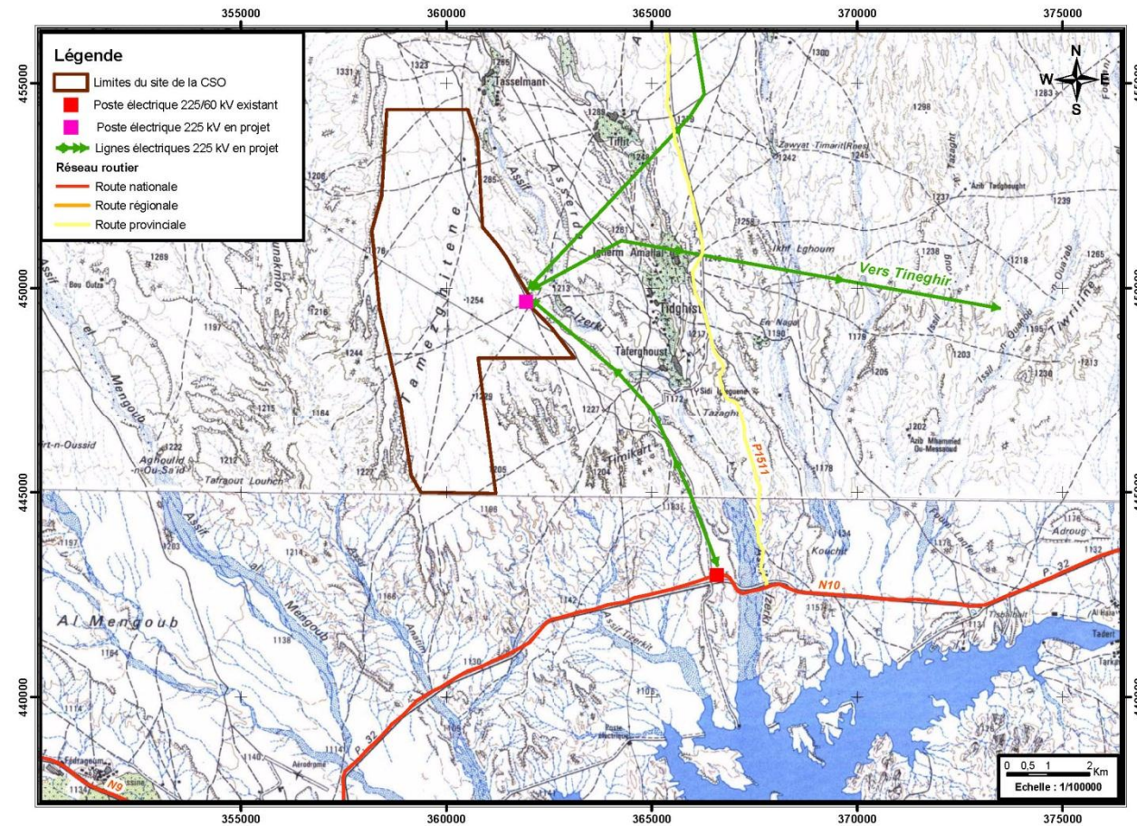
Figure 31 : Localisation du futur poste ONE 225kV au niveau du site et projection du couloir de la ligne de rabattement
